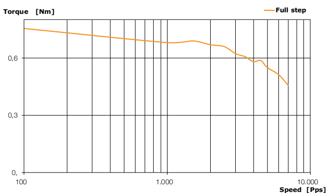
57STC41-2804AC VM: 24V; 2,8A/Phase Driver: SMD 103
